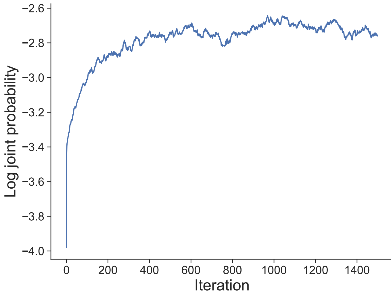
Dataset 16
