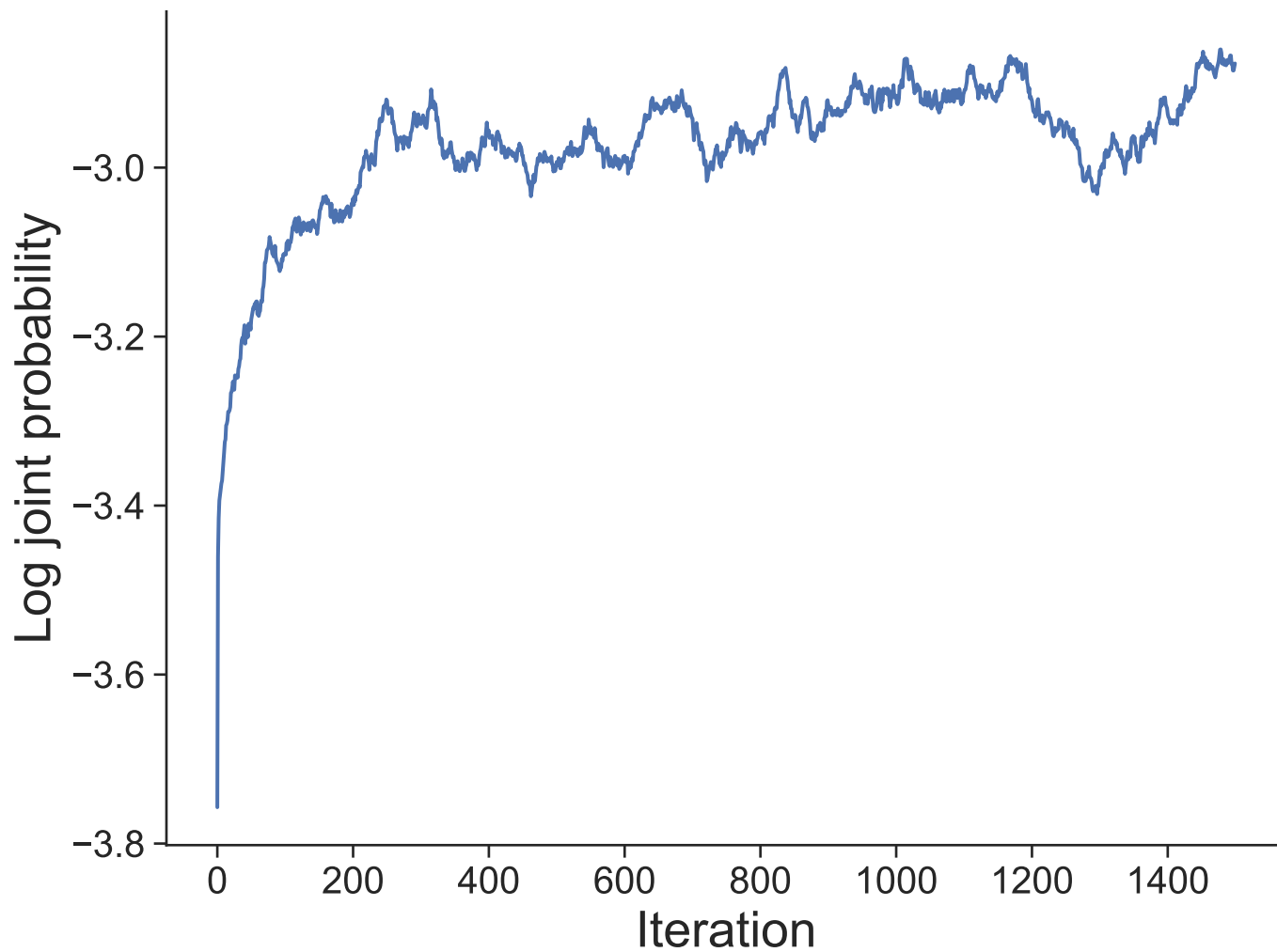
Dataset 21
