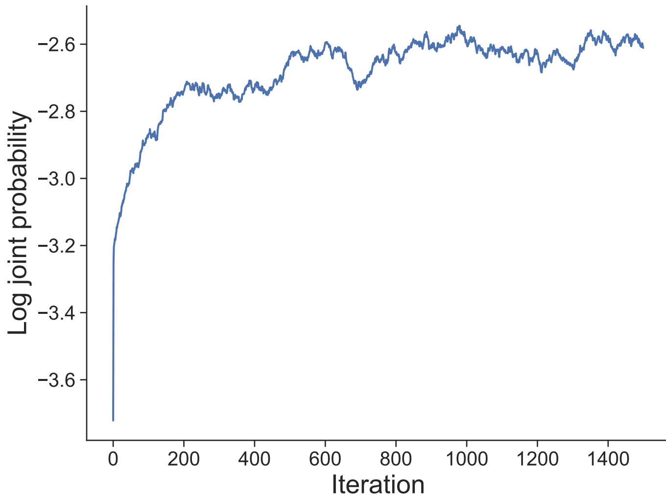
Dataset 39
