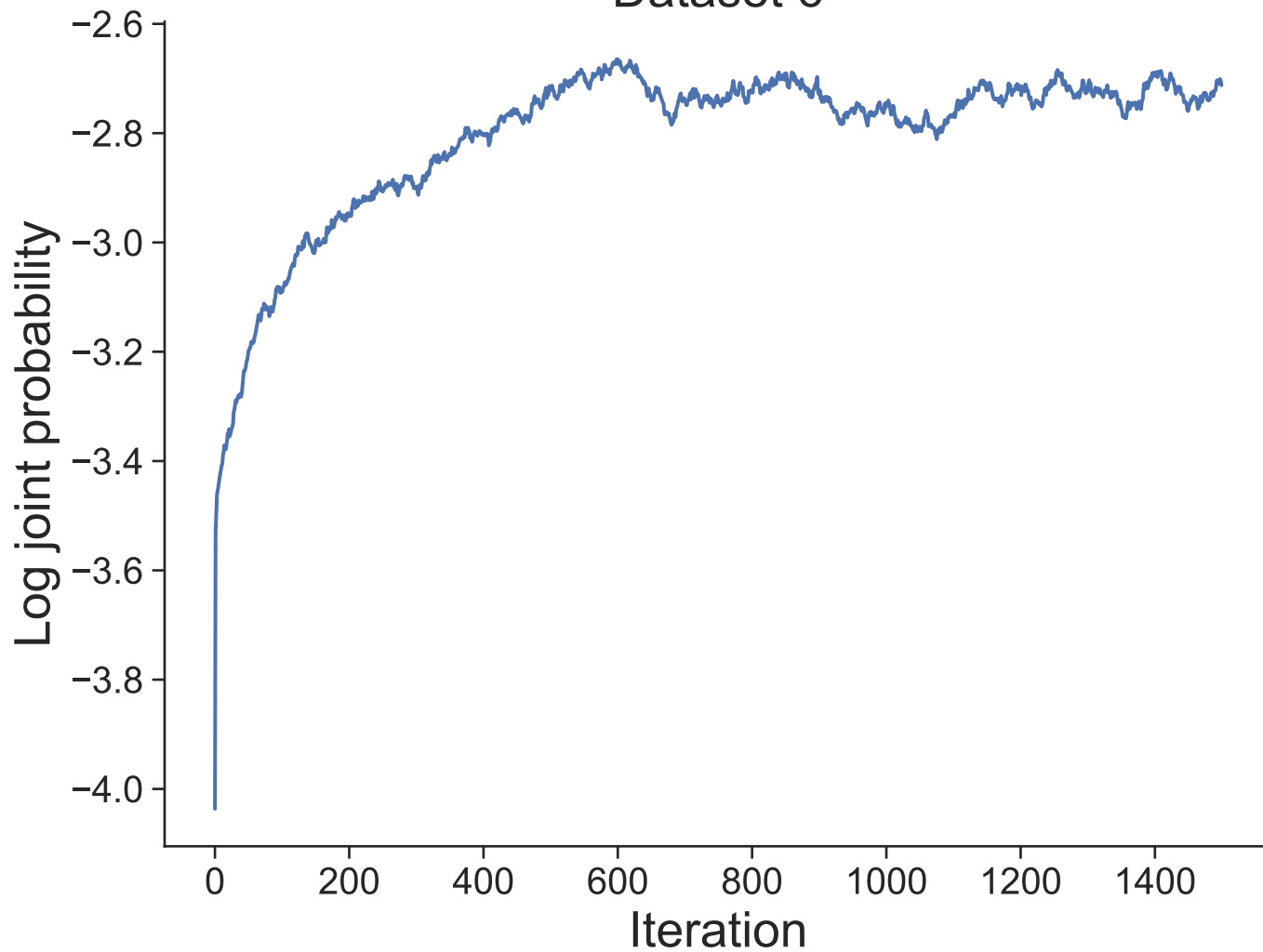
Dataset 6
