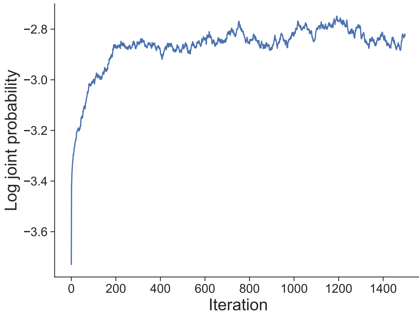
Dataset 15
