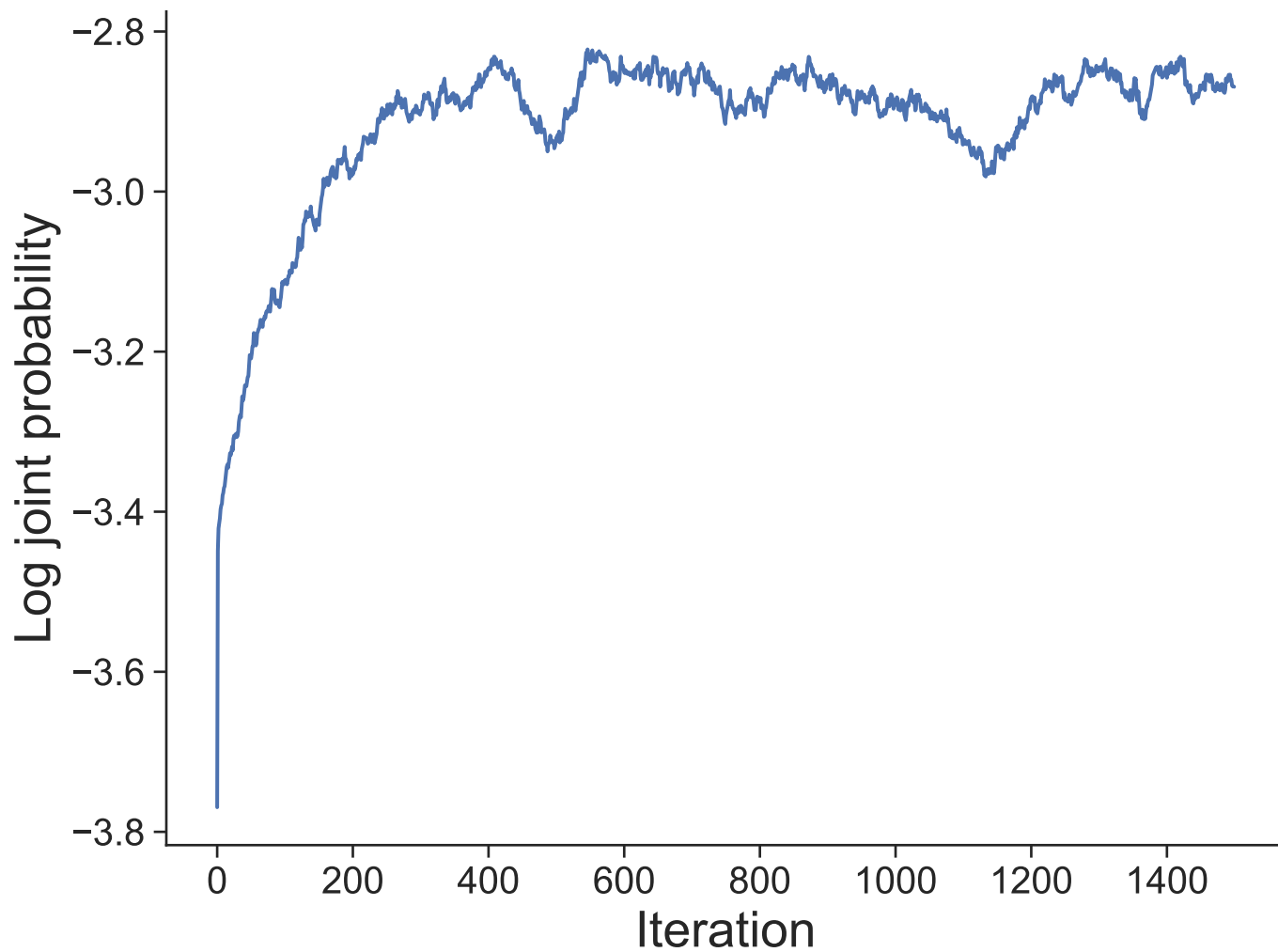
Dataset 48
