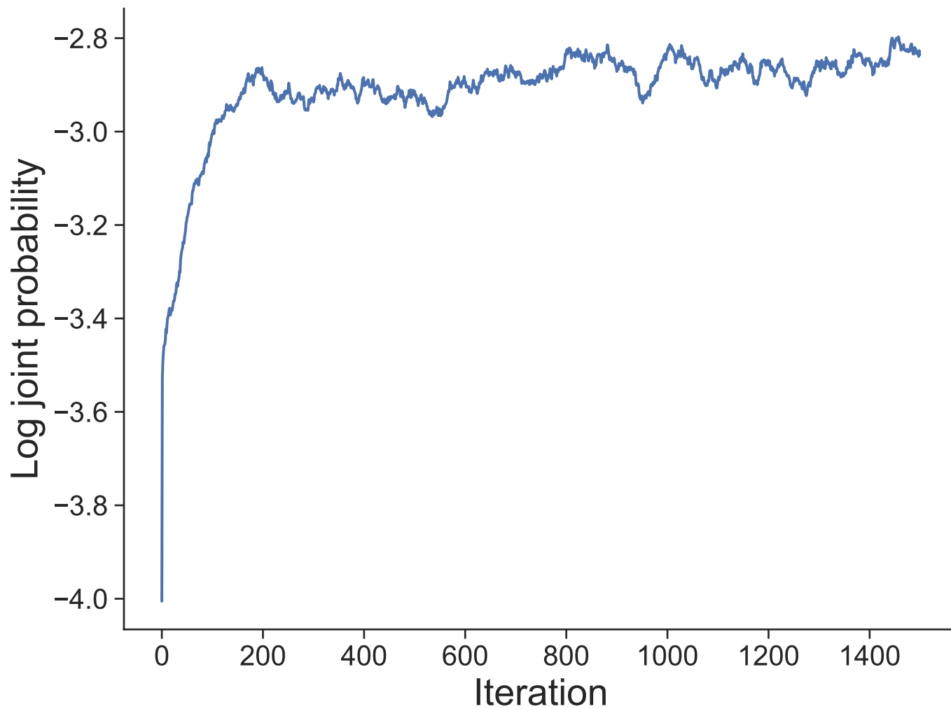
Dataset 27
