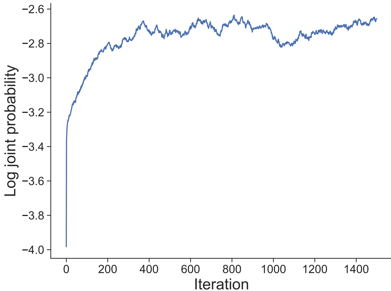
Dataset 28
