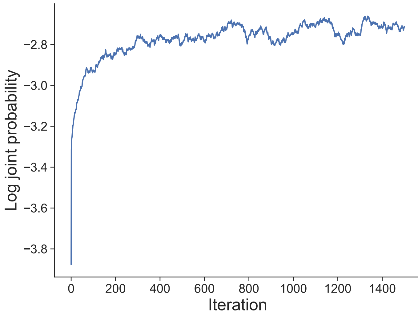
Dataset 40
