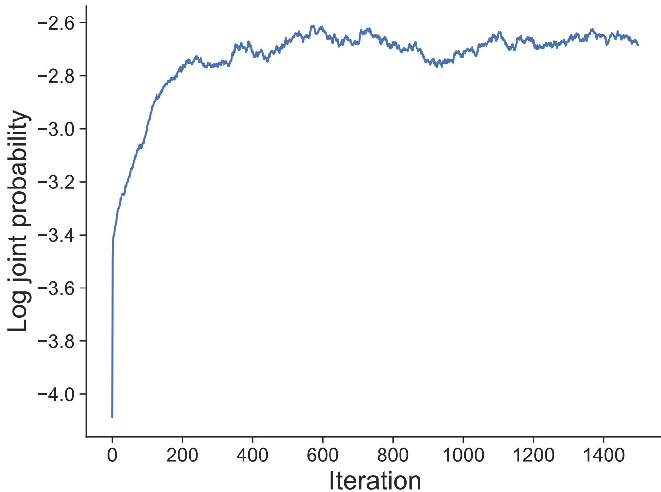
Dataset 47
