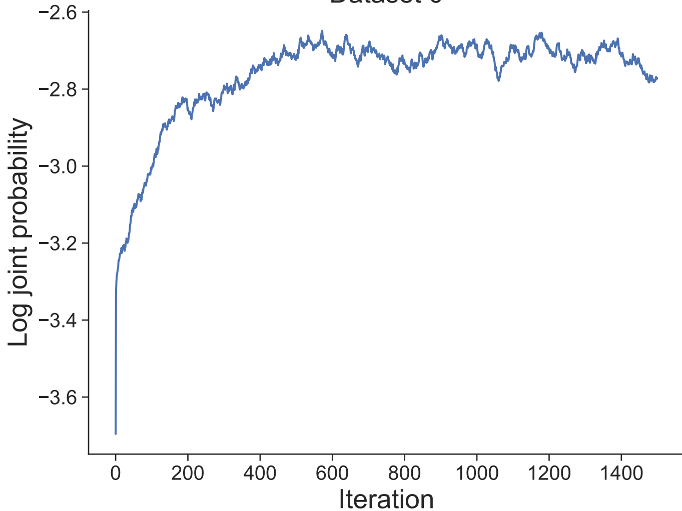
Dataset 0
