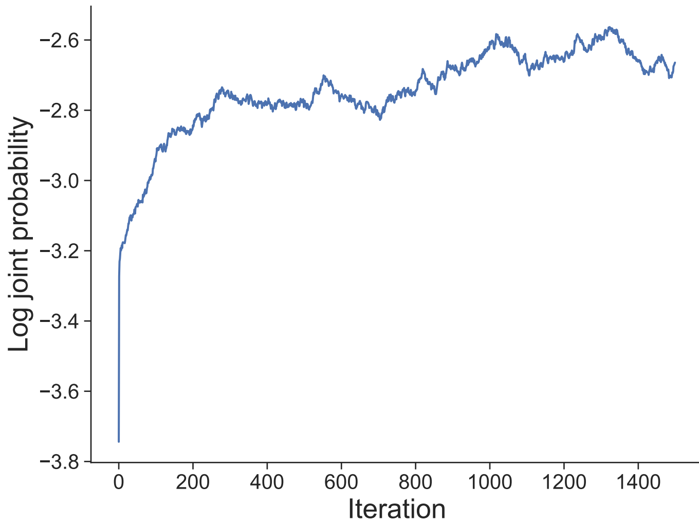
Dataset 23
