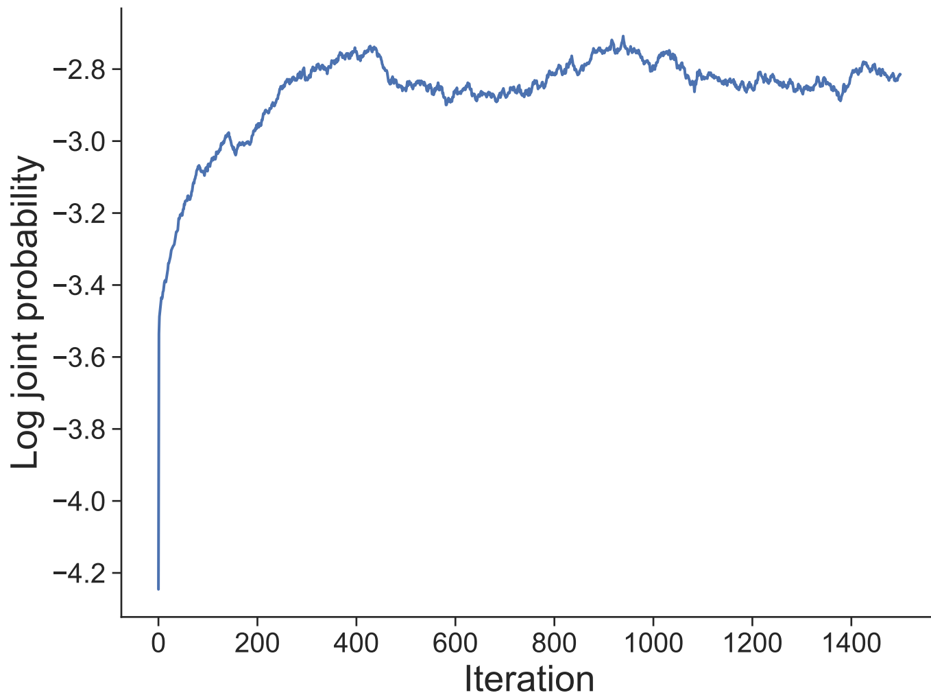
Dataset 31
