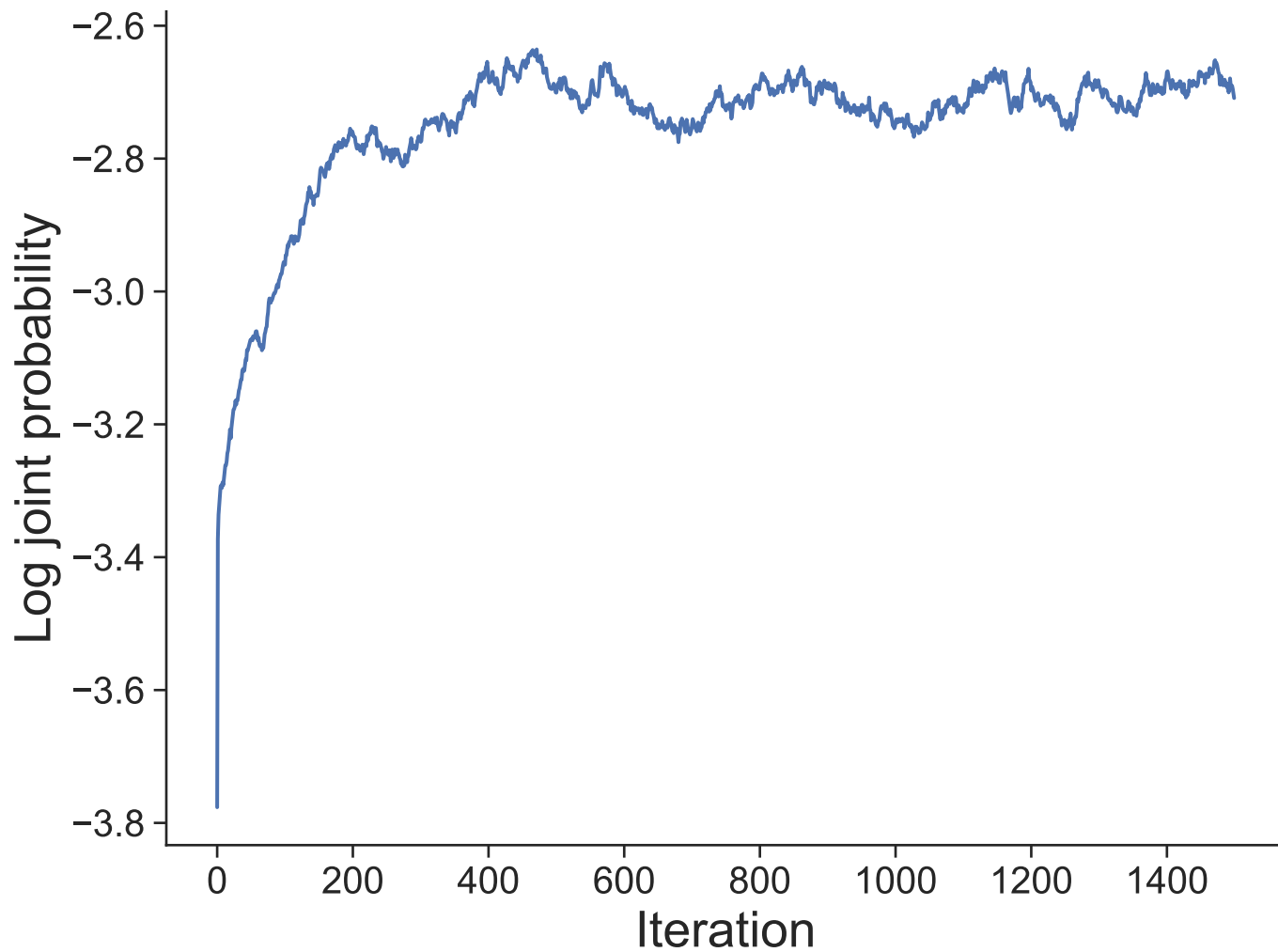
Dataset 22
