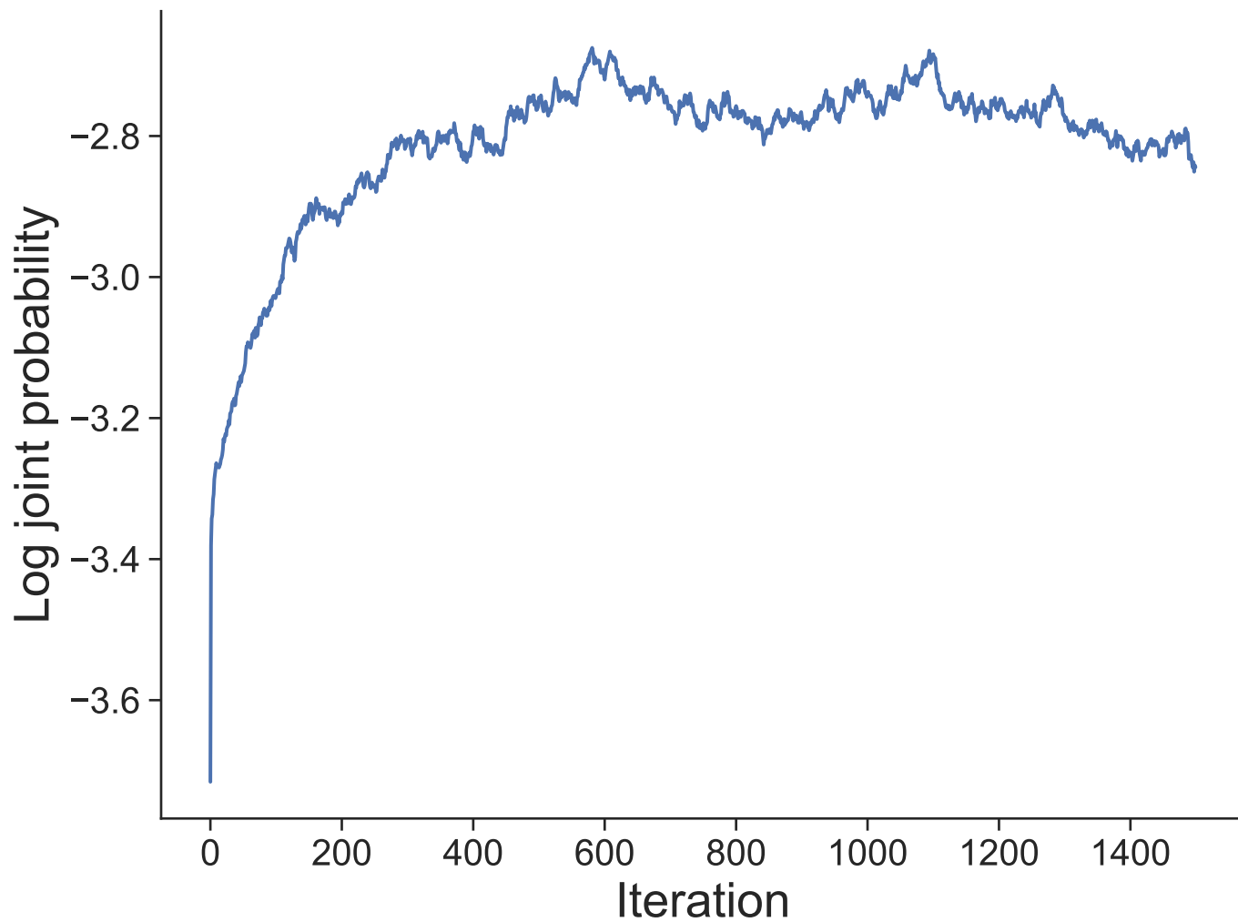
Dataset 32
