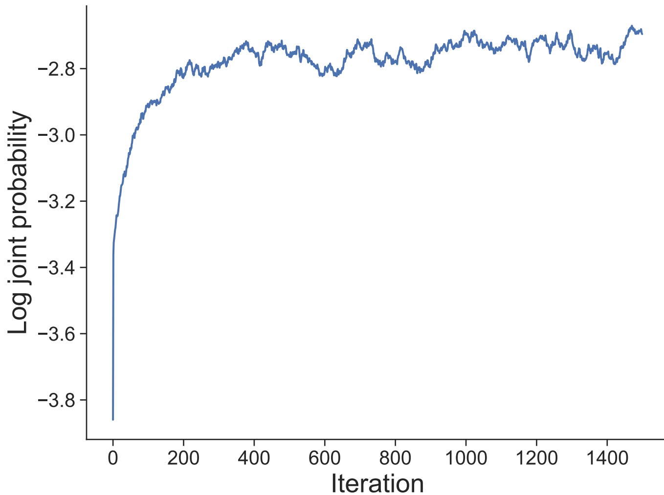
Dataset 5
