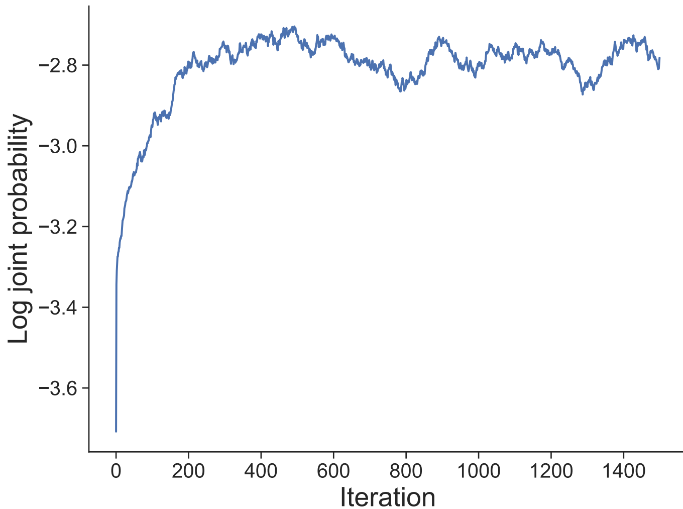
Dataset 19
