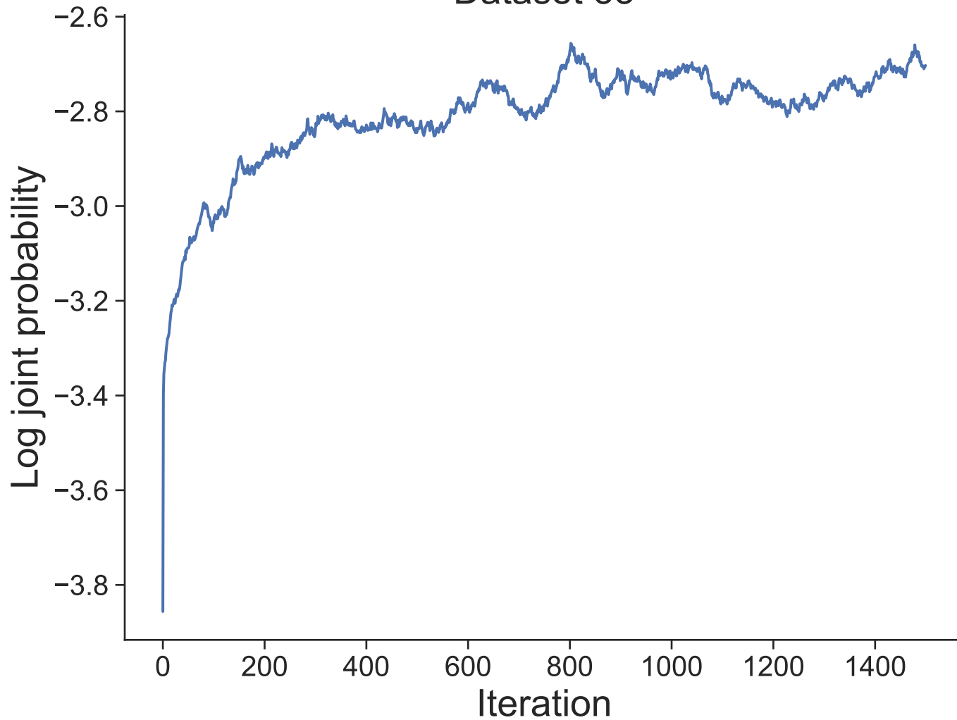
Dataset 33
