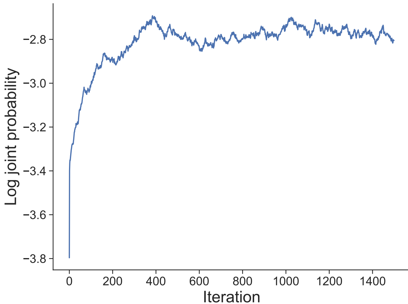
Dataset 26
