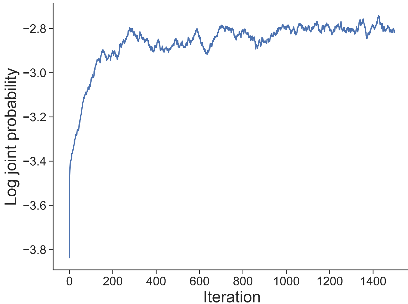
Dataset 38
