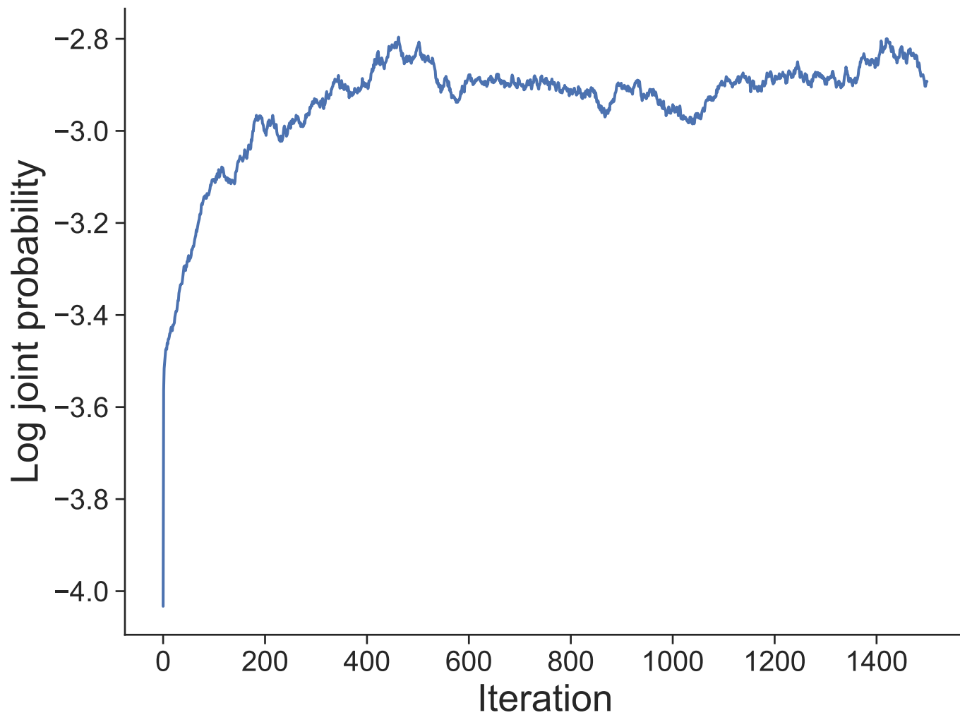
Dataset 37
