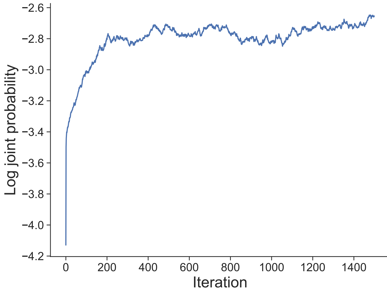
Dataset 24
