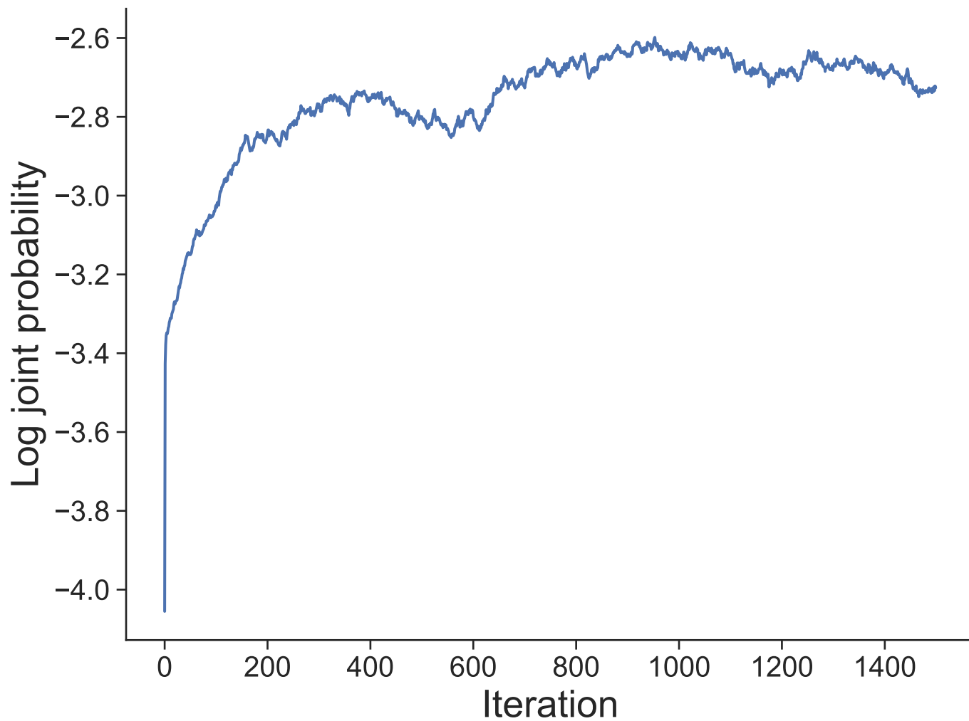
Dataset 2
