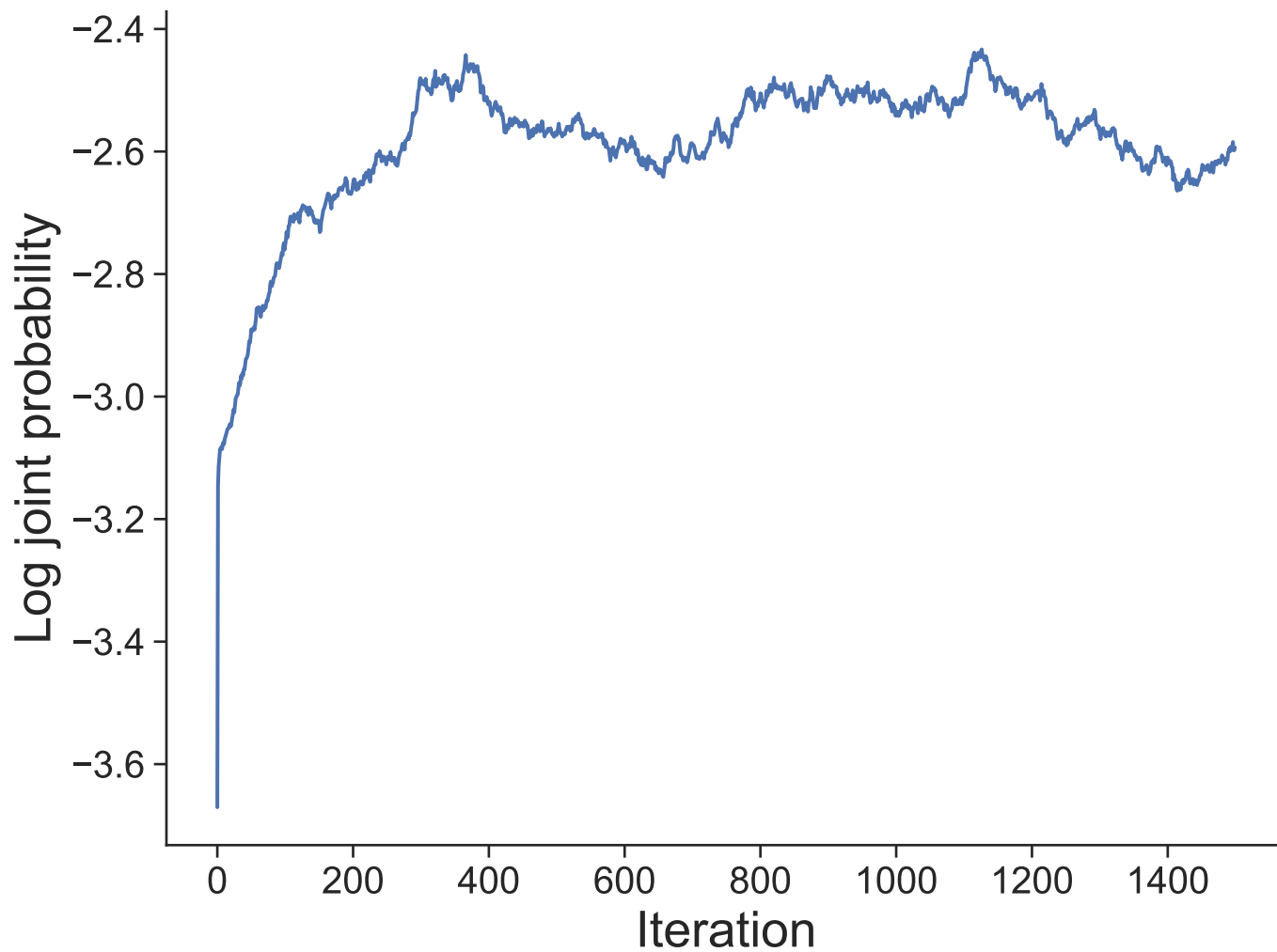
Dataset 45
