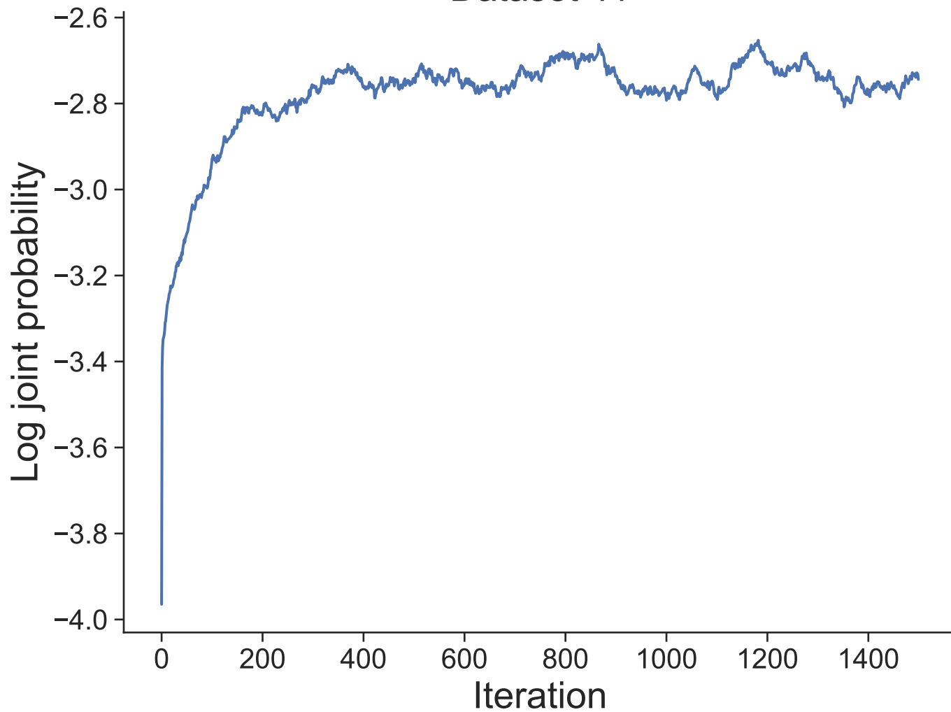
Dataset 41
