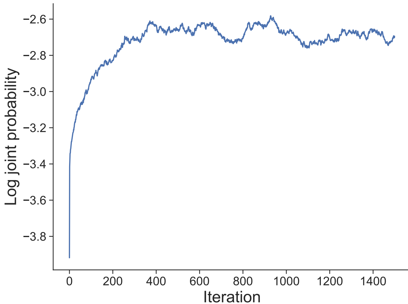
Dataset 20
