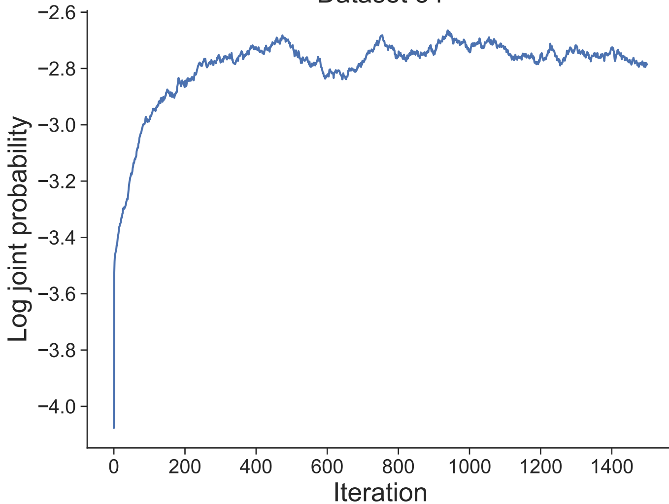
Dataset 34
