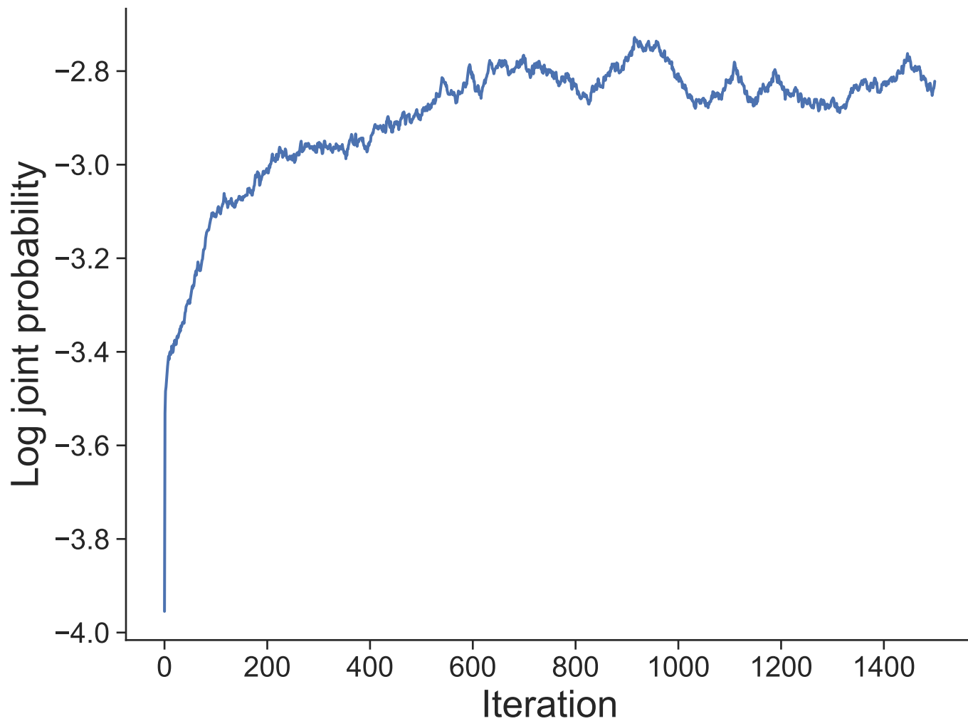
Dataset 12
