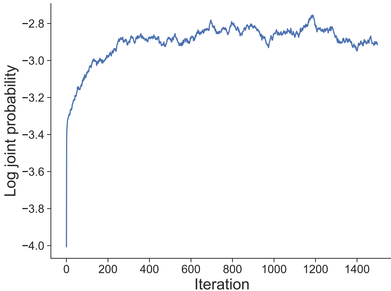
Dataset 10
