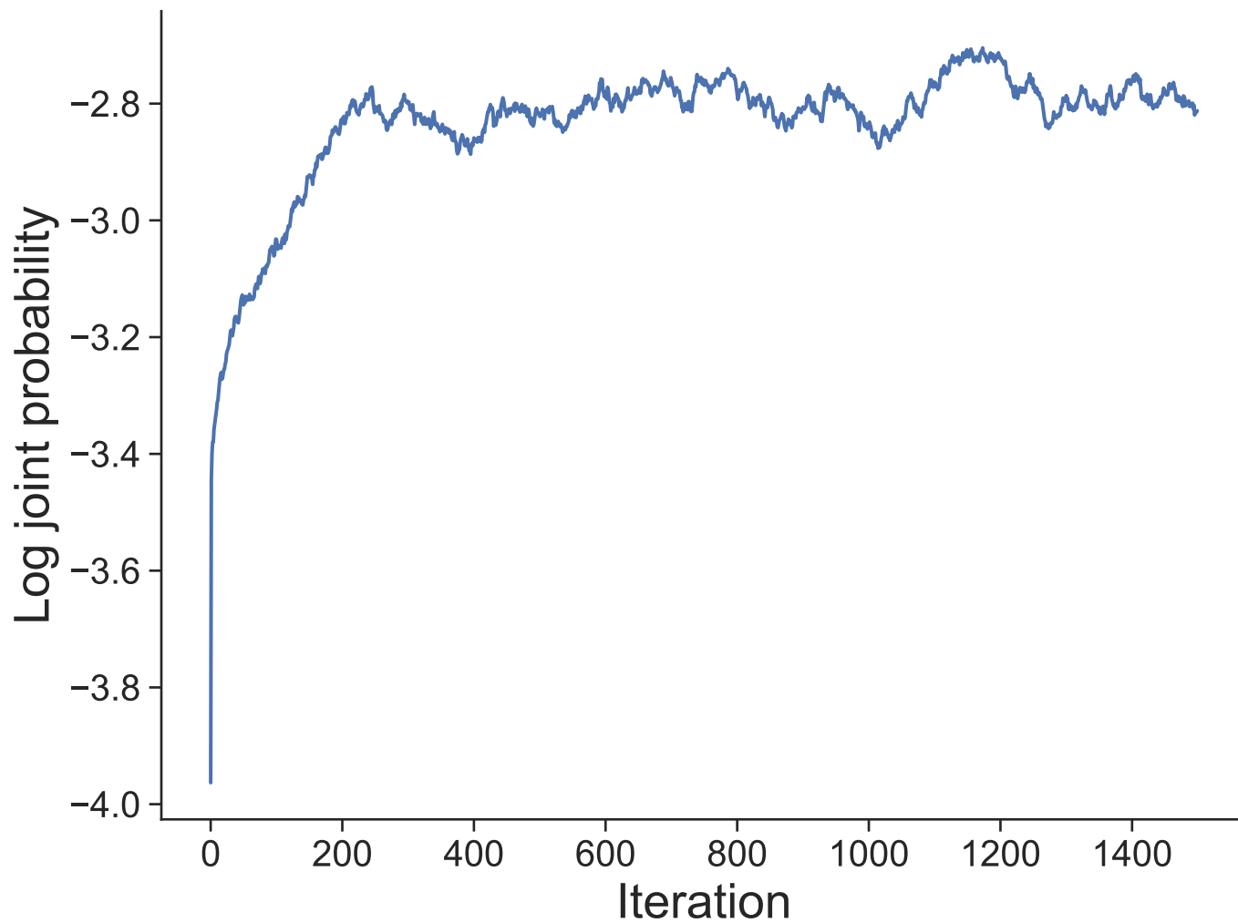
Dataset 42
