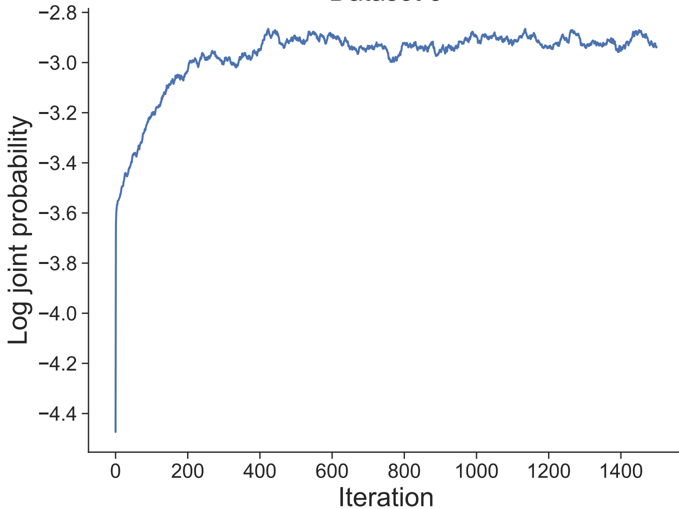
Dataset 3
